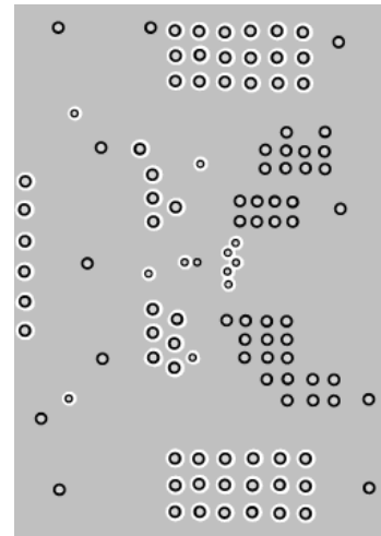
Inner Layer 1
