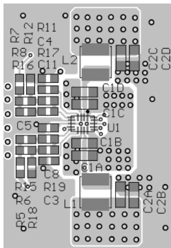
Top Layer
